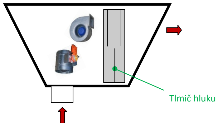
2. Strešná jednotka SJ s odhlučneným výtlakom vzduchu
