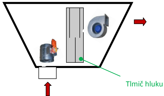
1. Strešná jednotka SJ s odhlučneným odvodom vzduchu
