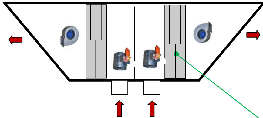
4. Strešná jednotka 2SJ s odhlúčeným odvodom vzduchu
